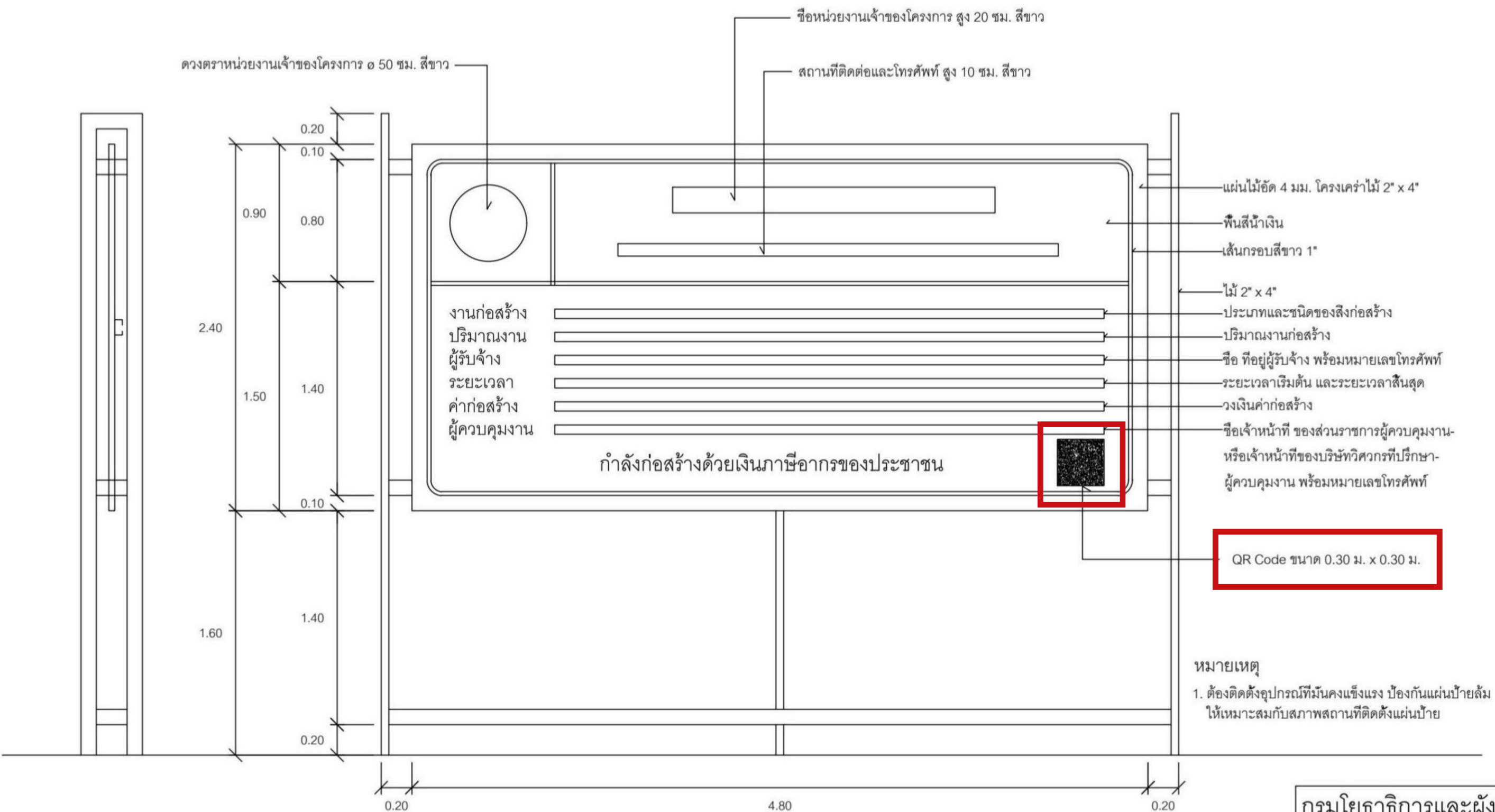
รูปด้านข้าง 1 : 25
